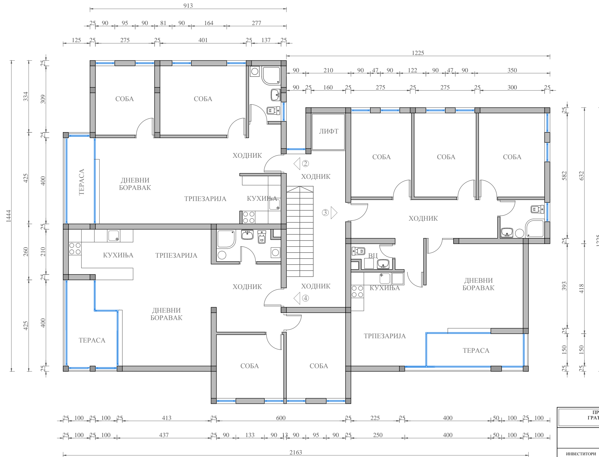
ОСНОВА ТИПСКОГ СПРАТА - ОД 1. ДО 3. ЕТАЖЕ СТАМБЕНОГ ОБЈЕКТА - P = 1:100
